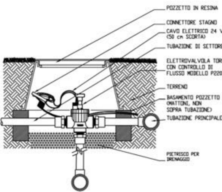
SCHEMA POSA POZZETTO 1:10
