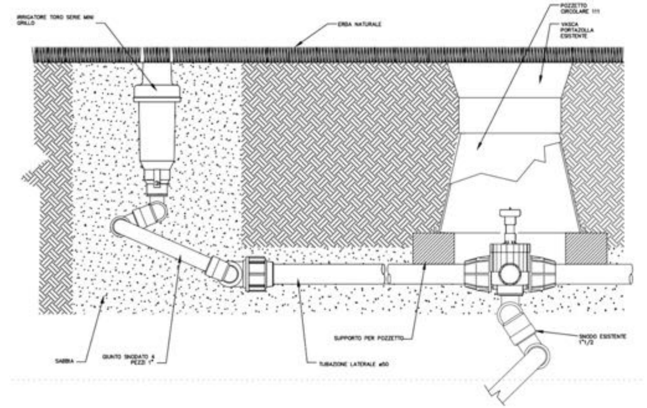
SCHEMA DI POSA IRRIGATORI - PER CAMPO IN ERBA NATURALE 1:10
