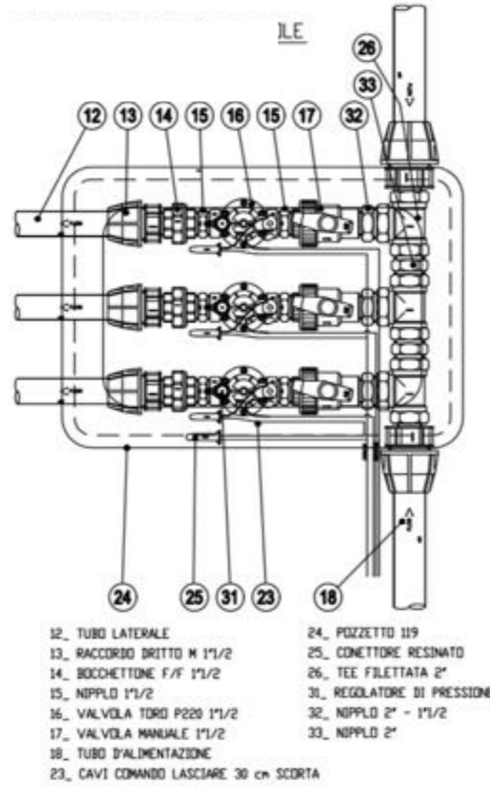
SCHEMA POSA POZZETTO VALVOLE 1:10
