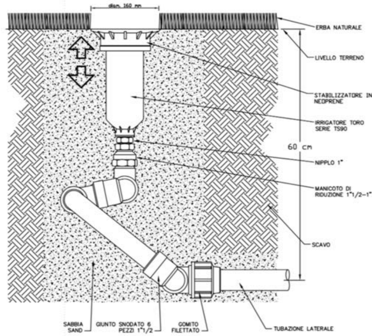
SCHEMA DI POSA IRRIGATORI PERIFERICI 1:10
