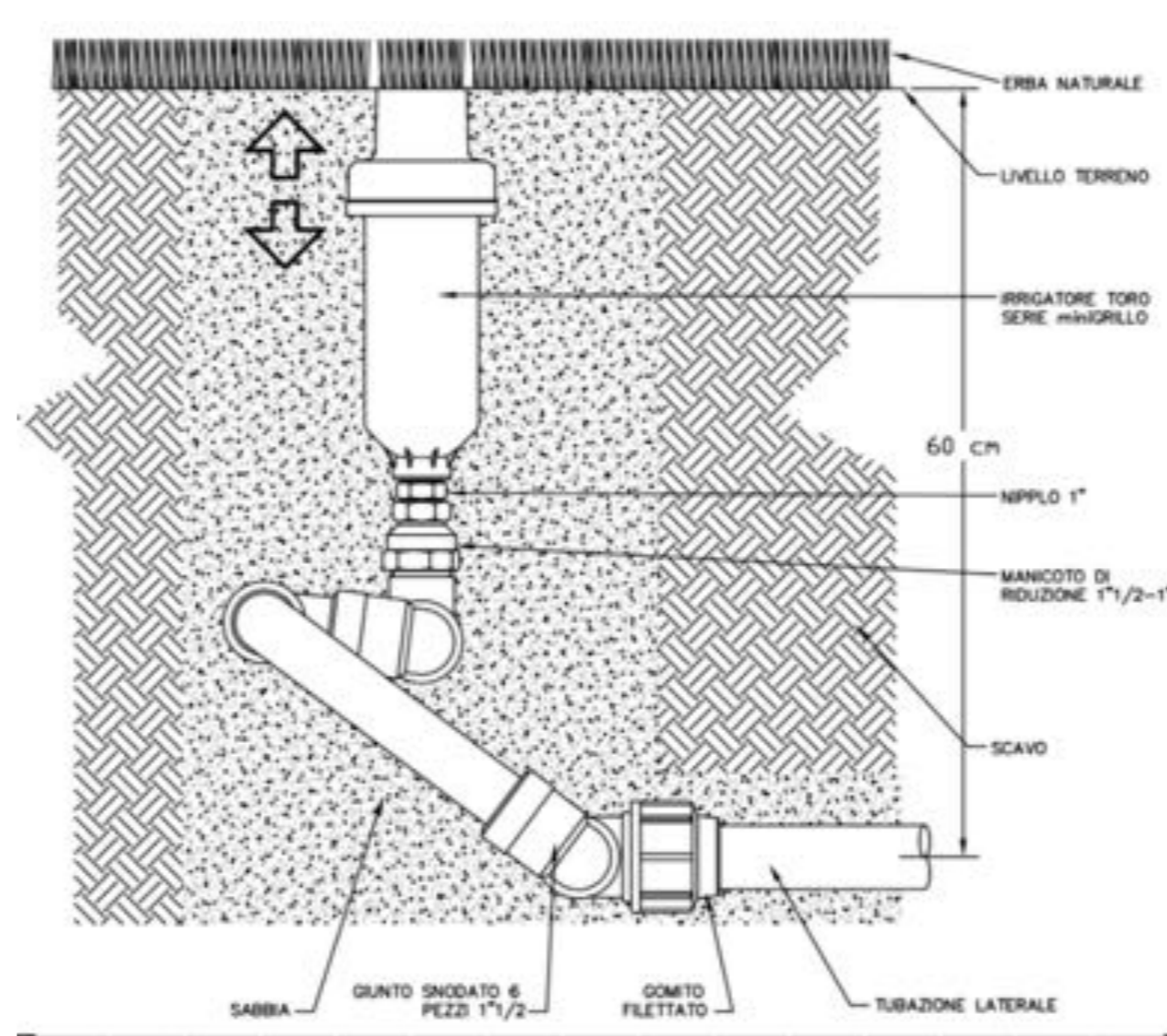
SCHEMA DI POSA IRRIGATORI CENTRALI 1:10
