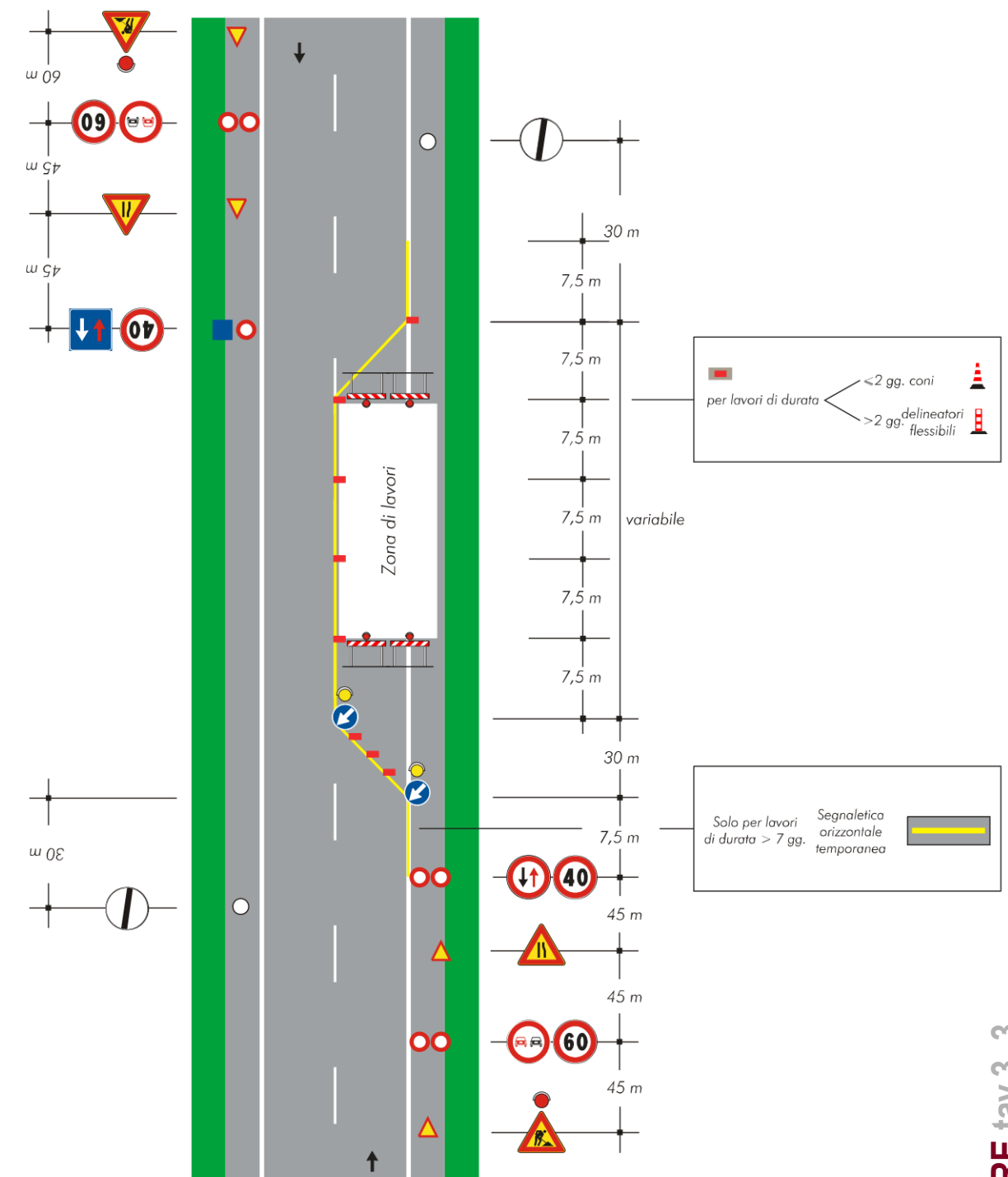
SCHEMA TIPO SEGNALETICA STRADALE (vedi disciplinare tecnico)
