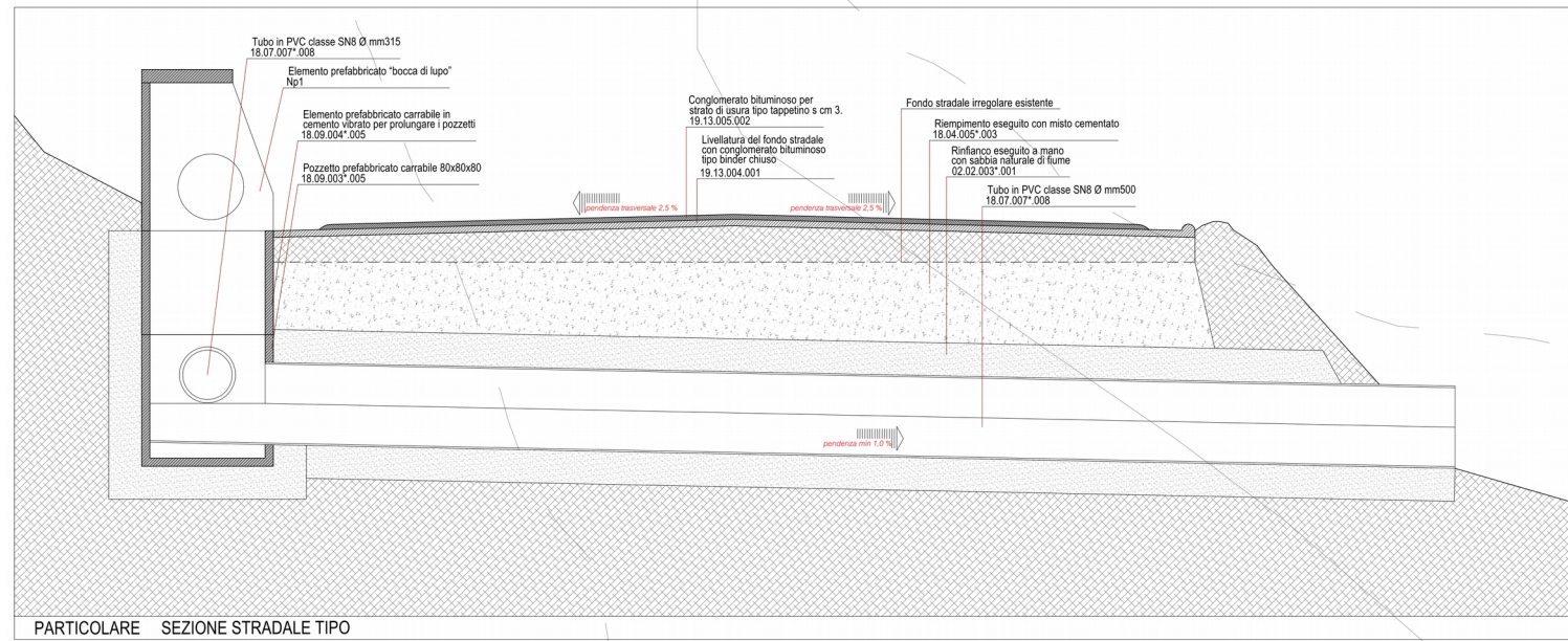
Schema tipo di intervento.
